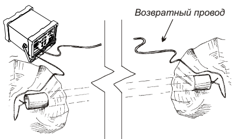
Гальваническое подключение с возвратом тока через провод
