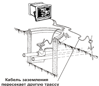
Нежелательное подключение
